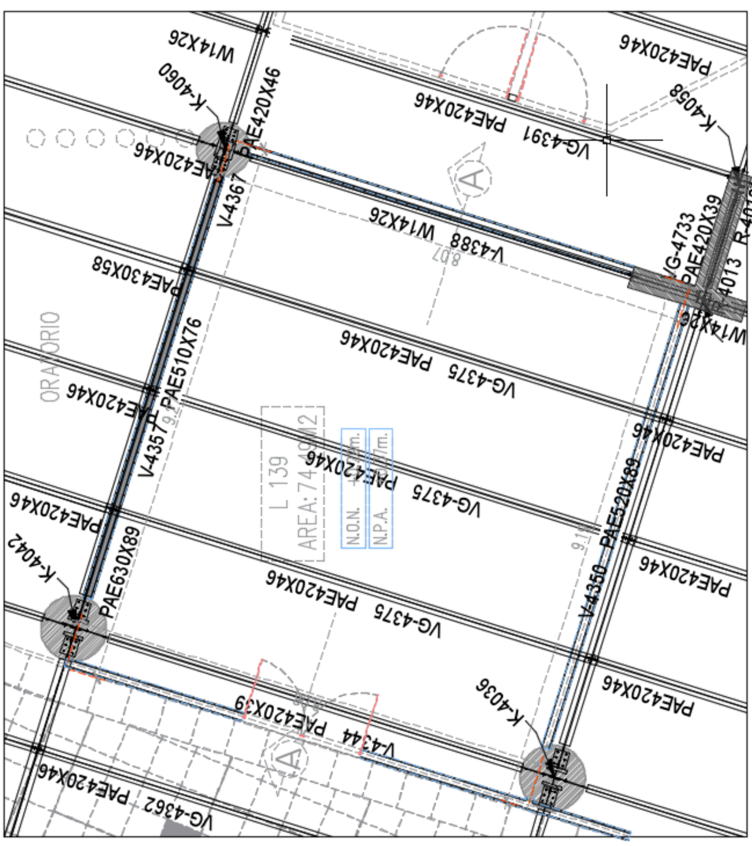
PLANTA PROYECCION DE CUBIERTA
