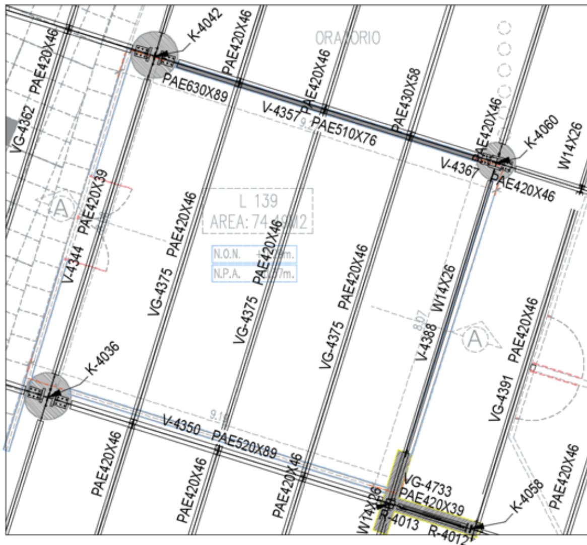
PLANTA PROYECCION DE CUBIERTA
