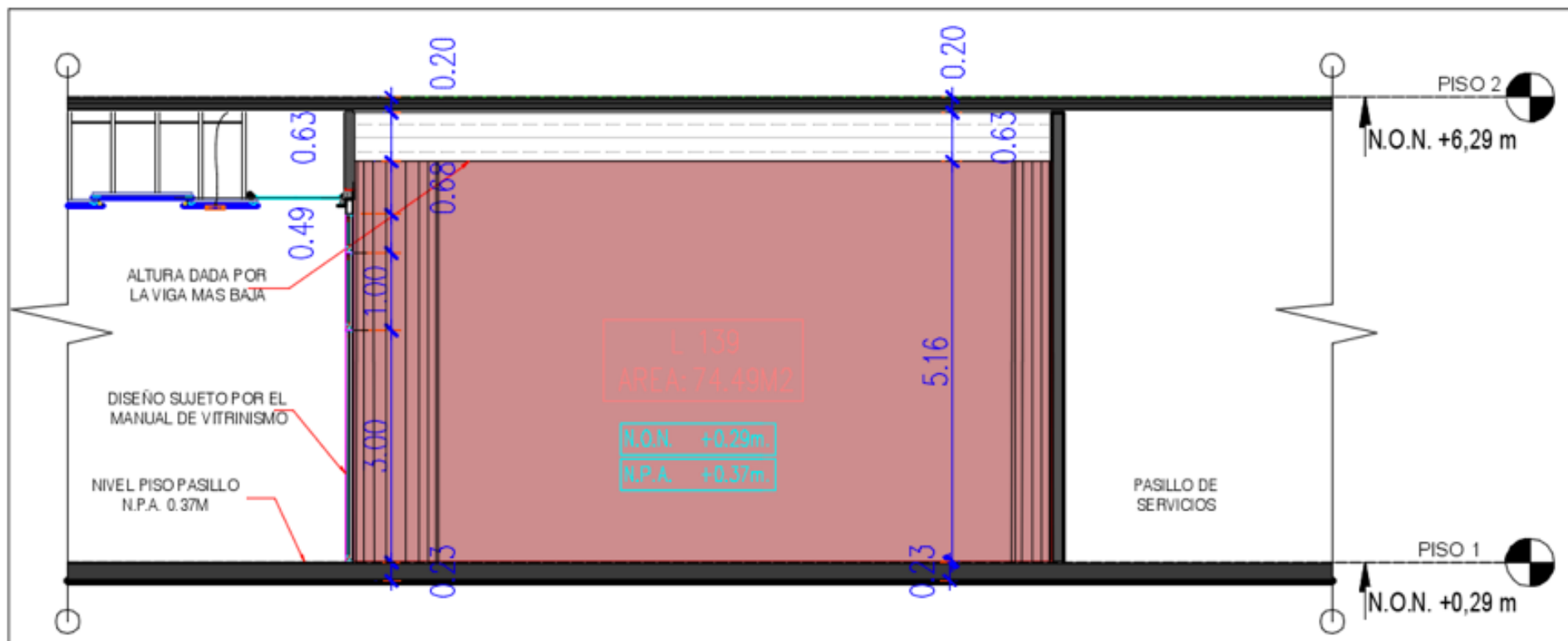
CORTE LONGITUDINAL A-A'
